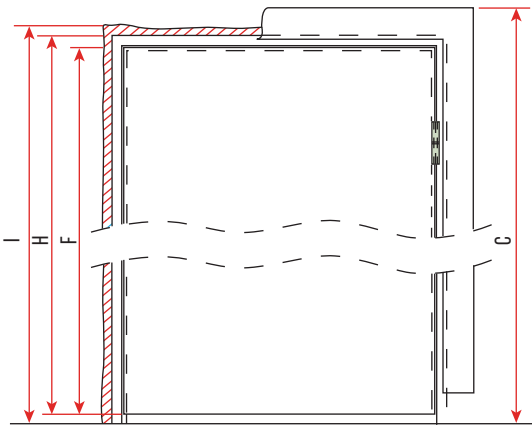
RESİM/PICTURE 2: KAPI YÜKSEKLİKLERİ/HEIGHT OF DOOR
