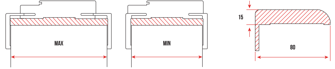
Pervaz Çalışma Payları/Frame Working Margins (0-60 mm)
