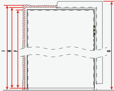
RESİM/PICTURE 2: KAPI YÜKSEKLİKLERİ/HEIGHT OF DOOR
